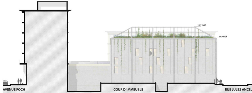
FAÇADE EST AU 1/200
