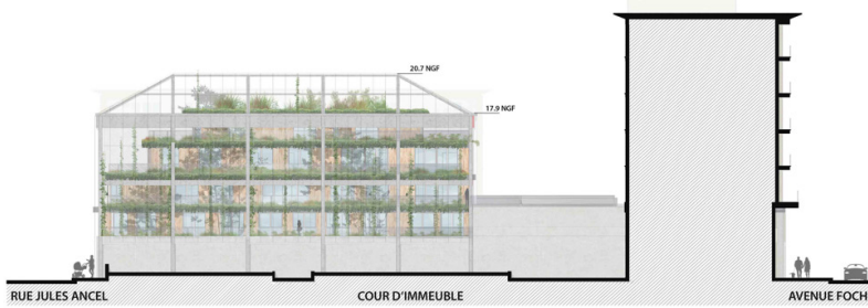
FAÇADE OUEST AU 1/200
